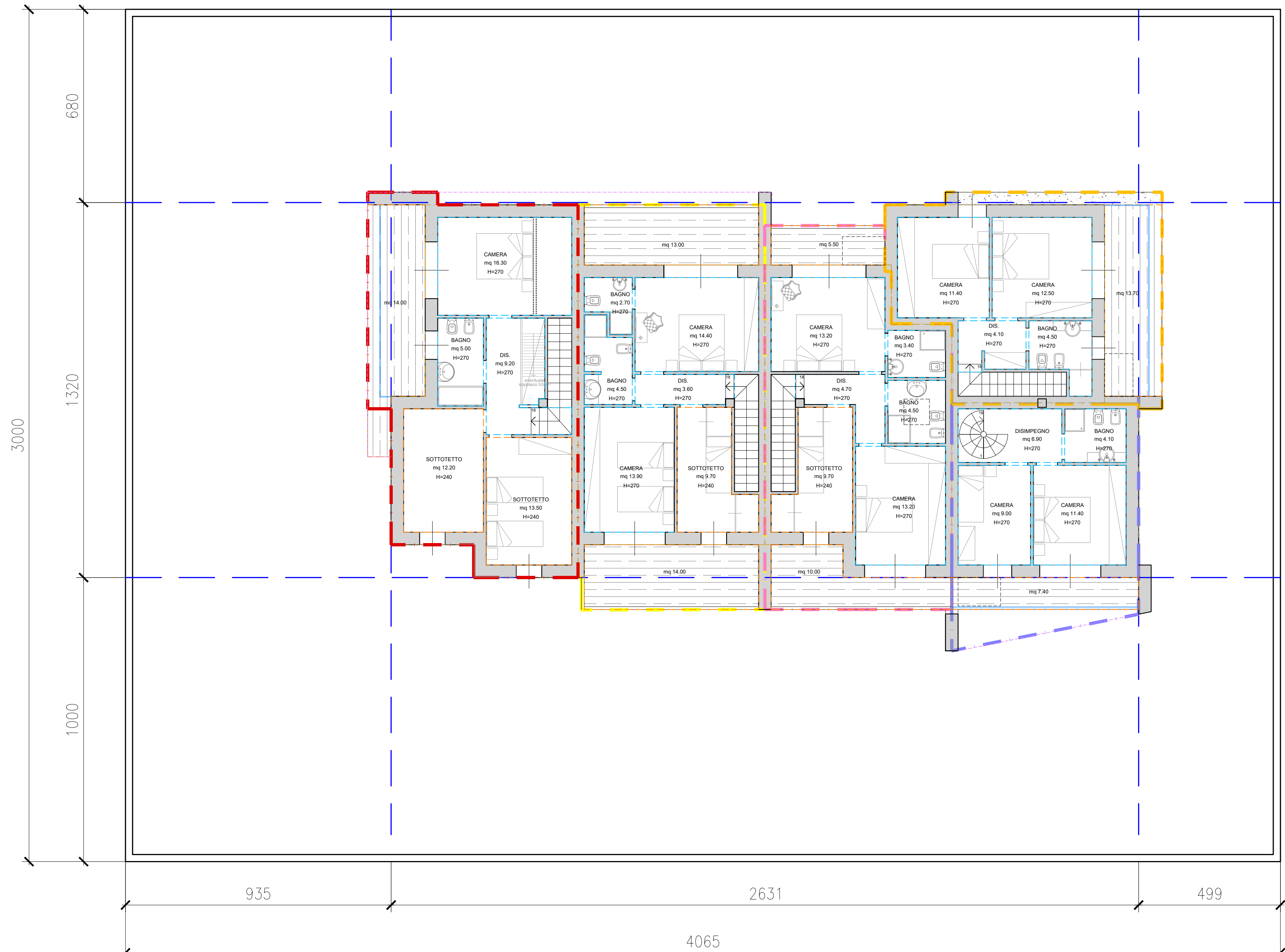
PIANO PRIMO
